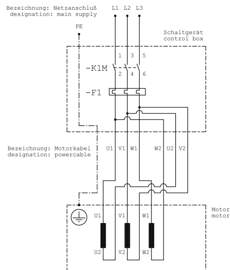
Abb. 3 / Fig. 3: Netzanschluss Direkt-Start (DOL) für Stern-Dreieck-vorbereitet Motoren (alle Wicklungsenden über Anschlusskabel zugänglich). Dreieckschaltung der Wicklung Starter connection Direct-on-line Start for Star-Delta Start prepared motors. Delta connection of stator windings
