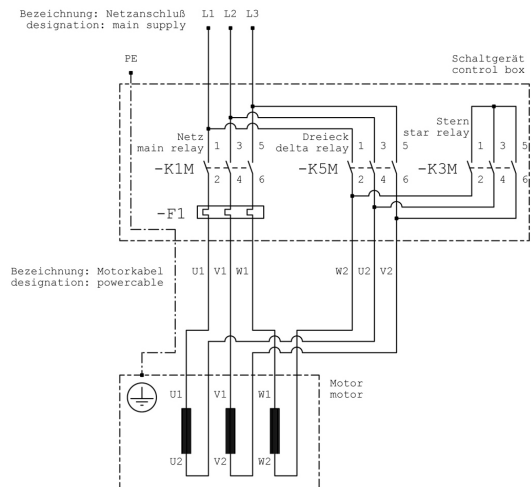
Abb. 2 / Fig. 2: Netzanschluss Stern-Dreieck Starter connection Start-Delta Start
